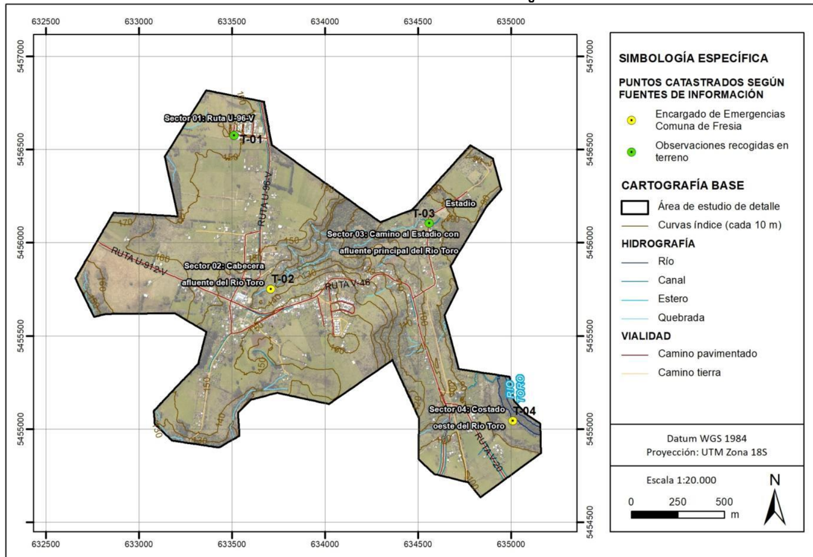
FIGURA Nº 4-2 Mapa de catastro de eventos de inundación por desborde de cauce y anegamiento con información recogida durante la campaña de terreno en el área de estudio de detalle de Tegualda.
